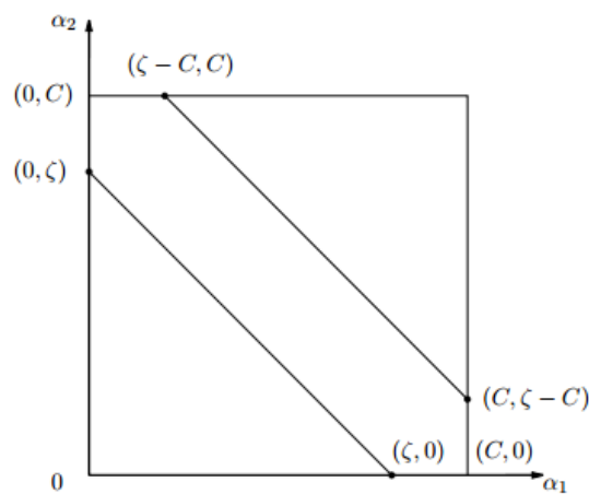
图 18: SMO 算法情况 2
